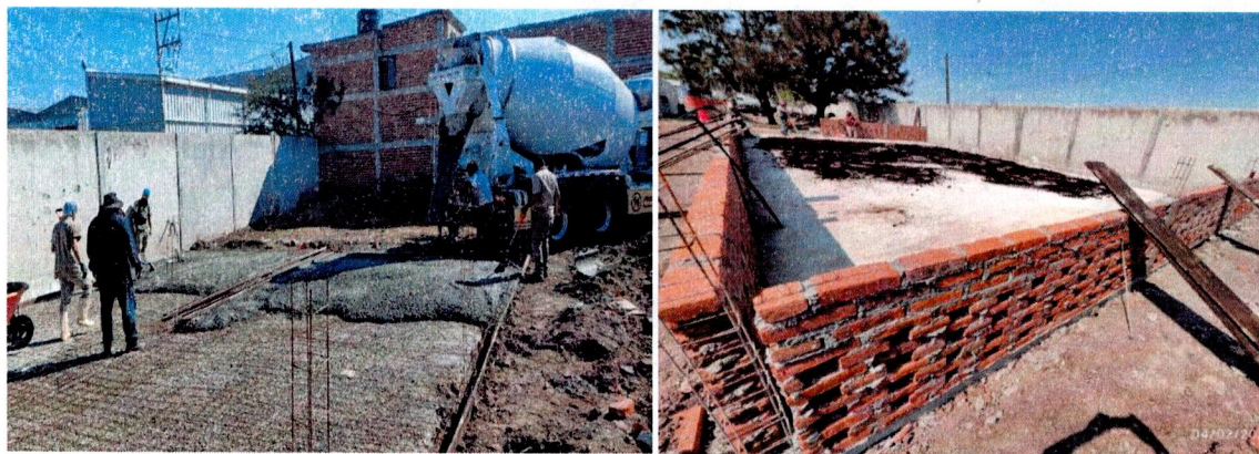
Figura 9. Construcción plancha de secado. Fuente: Informes mensuales de enero-marzo 2026 de la Dirección de Rastro
