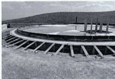
OBRA_20_JAPAMI-LPN-RP-2024-29 Construcción de Tanque de Vidrio Fusionado al acero en la Zona Alta de Villas de Irapuato.
